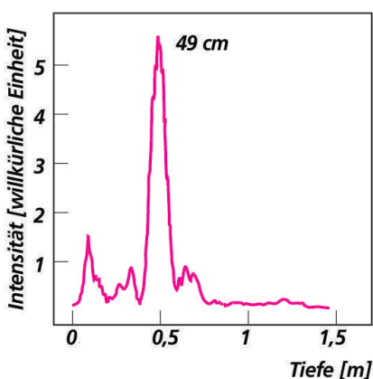
Abb. 7 Bestimmung der Dicke einer Betonplatte, die in 50 cm Tiefe ein reflektierendes Element (Arbeitsfuge) enthält: Tiefenverteilung der rückgestreuten Ultraschall-Energie (nach [3, 10]).
