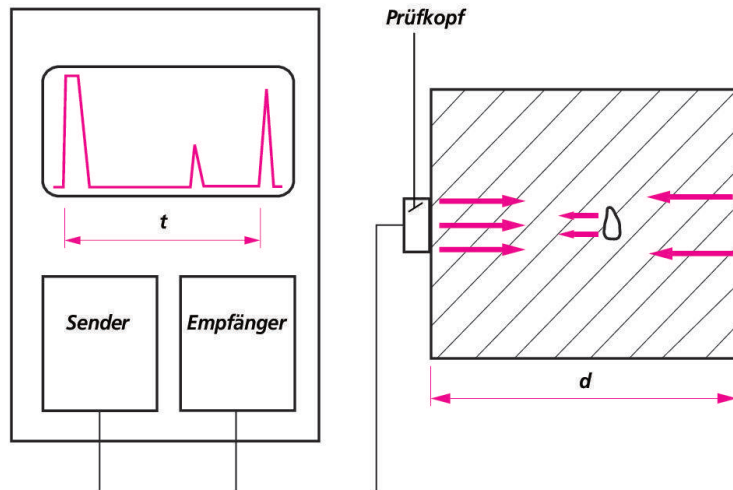
Abb. 6 Schematische Darstellung einer Ultraschall-Impuls-Echo-Messung (nach [9]).
