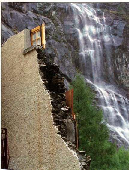
La ruine de la mairie de Gondo après le glissement de terrain d'octobre 2000.
