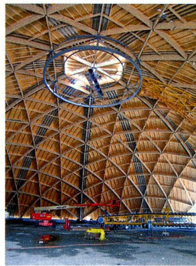
Riburg, 2005: centre logistique et de stockage des salines du Rhin avec une coupole en bois haute de 31 mètres.
