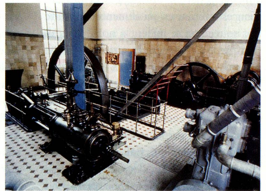
Uster, 1980: cuves de brassage de la brasserie d'Uster, avec la dernière machine à vapeur de l'Oberland zurichois. La machine de ventilation et un compresseur de refroidissement datent de 1897.
