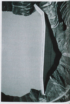
Barrage de la Grande-Dixence dans le val d'Hérens, 1968
