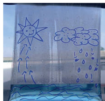
Ciclo hidrológico
