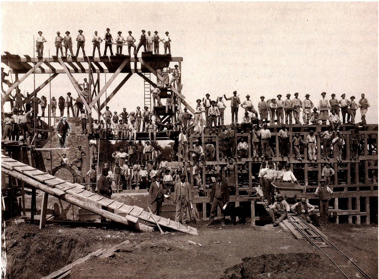
Fábrica mecánica de tejas y ladrillos en Allschwil, fotografiada en torno a 1898
