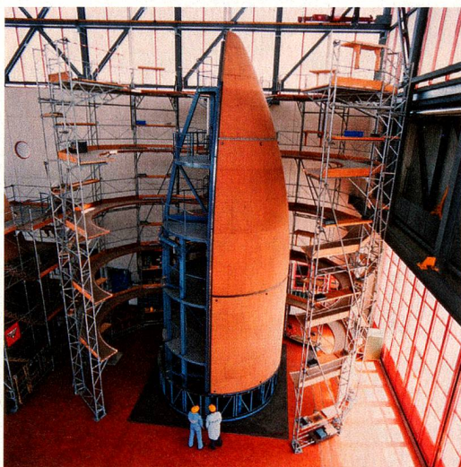
Construcción de cohetes en Emmen, fotografiada en torno a 1992
