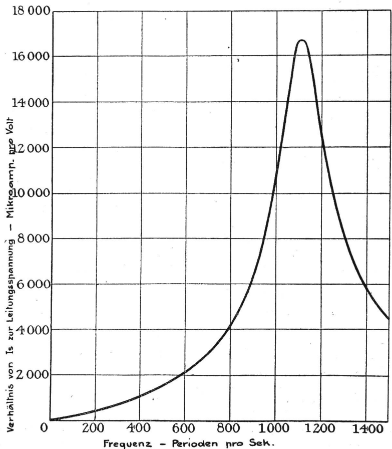
Fig. 8. Schaltschema und Eichkurve des Telephonstörungsfaktormessers der Spannungswelle.
