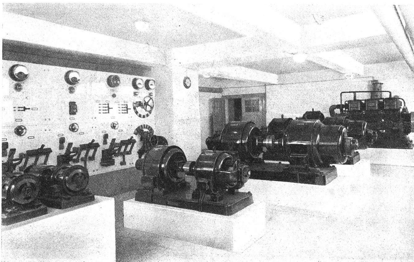
Fig. 18. Kraftanlage.
