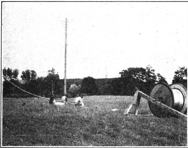
Abb. 4. Kabelhaspel aufgebänkt.
