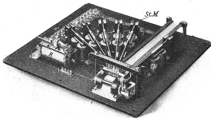
Fig. 5. Oberteil des Lochers. — Partie supérieure du perforateur.
