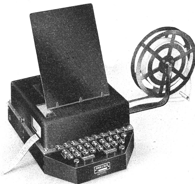
Fig. 4. Lochapparat. — Perforateur.
