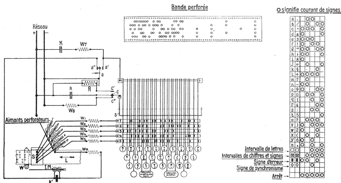
Fig. 1. Schaltbild des Lochers, Lochstreifen und Zeichentabelle.
