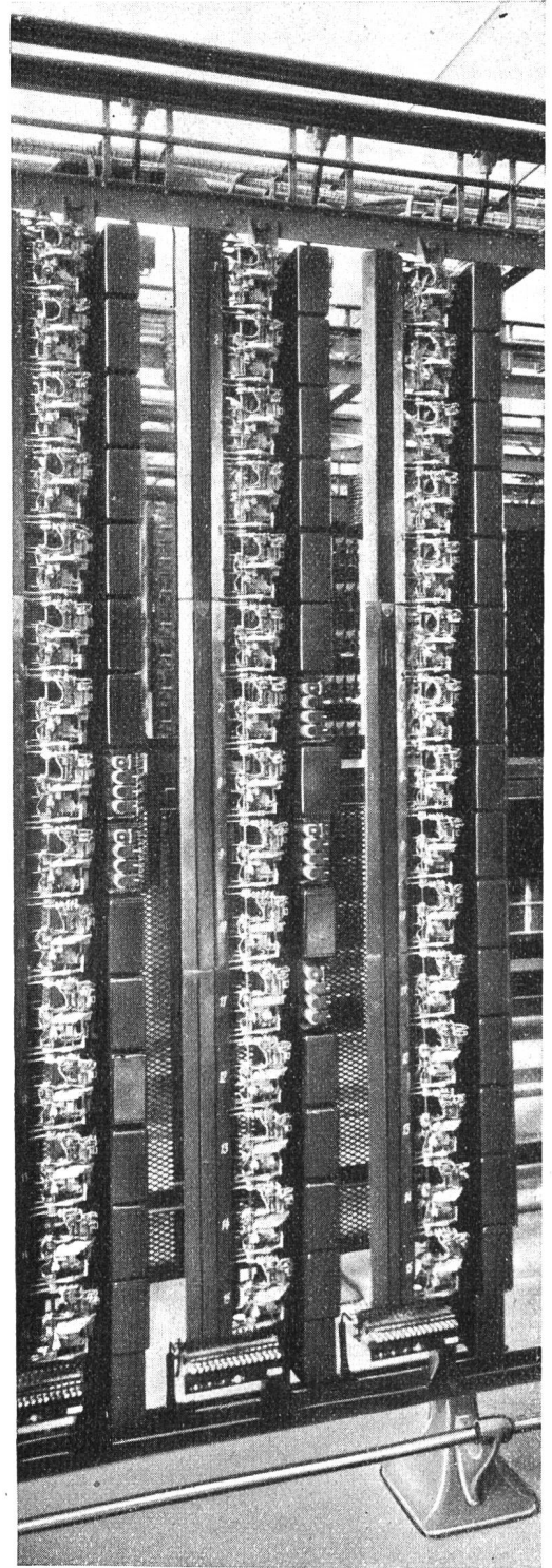
Fig. 8. Wählerrahmen.
