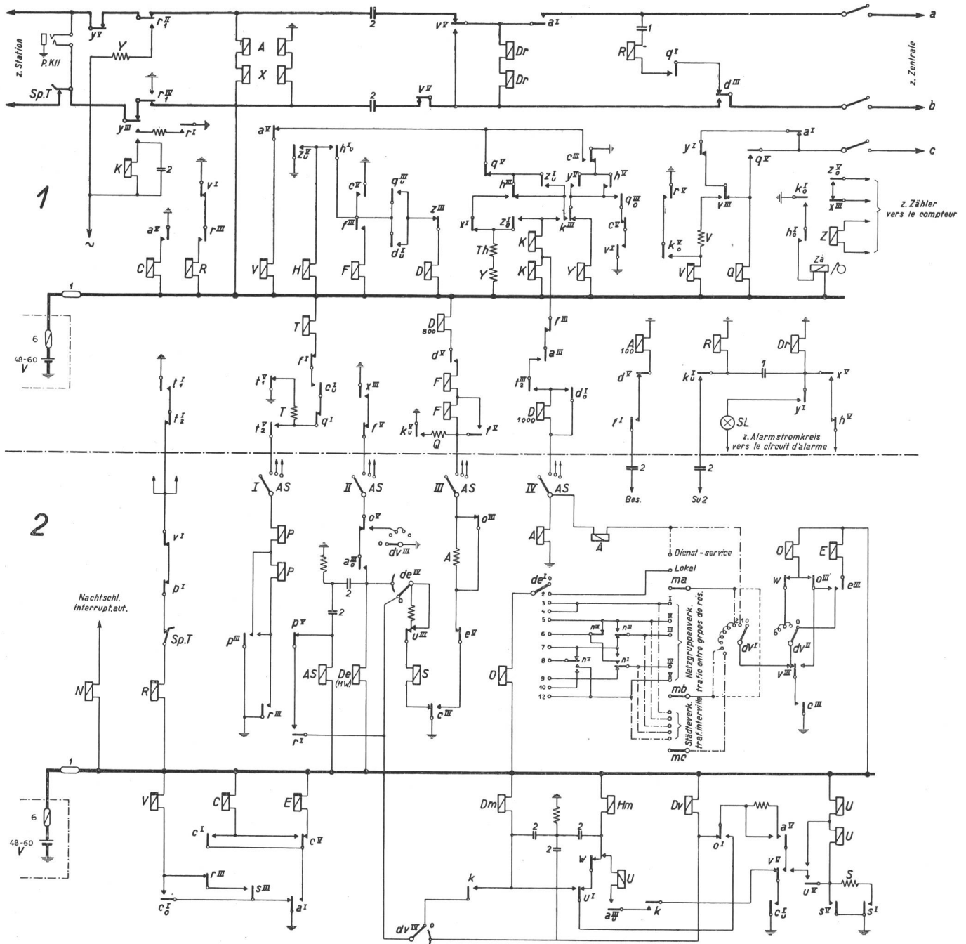
Fig. 13. Zusatzschaltung für vollautomatischen Orts- und Fernverkehr mit gemeinsamen Münz- und Zonenschaltern.
