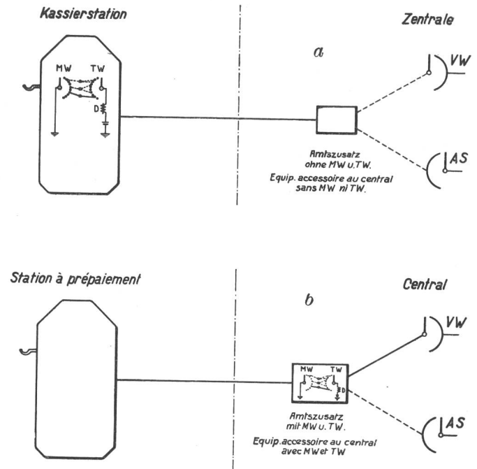
Fig. 2a. Münz- und Taxwähler in der Kassierstation untergebracht.
