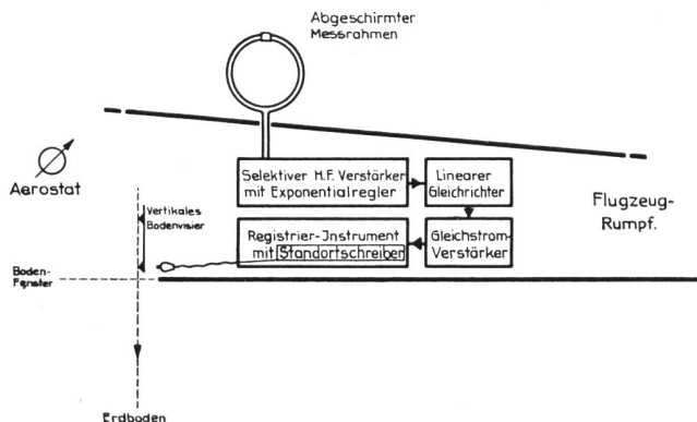
Fig. 3. Flugzeugausrüstung zur Aufnahme vertikaler Strahlungsdiagramme.
