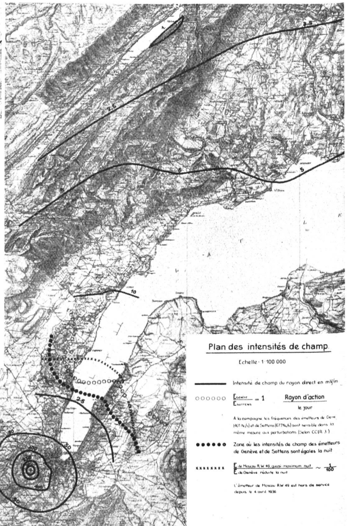
Fig. 16. Feldstärkenplan. Landessender Sottens. 100 kW; 677 kc/s.
