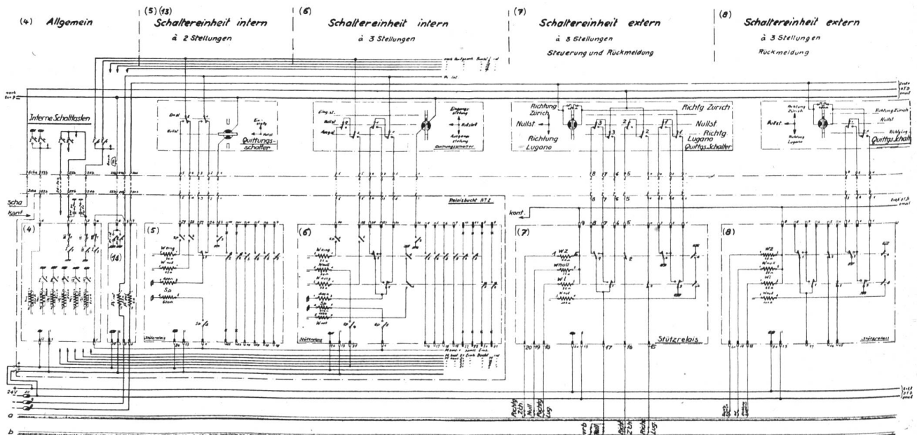
Abb. 3. Schaltung der Schaltereinheiten des Senders, sowie der internen Steuerung der Rundfunkverstärker in Zürich.
