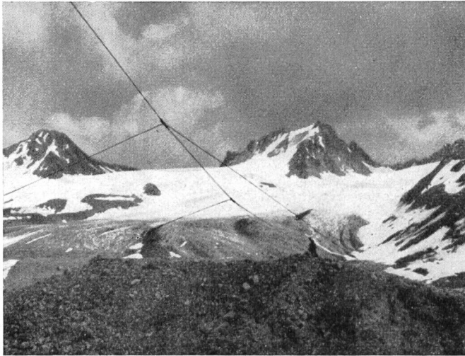
Abb. 4. An Felswand befestigte Queraufhängung der Leitung nach der Keschhütte.
