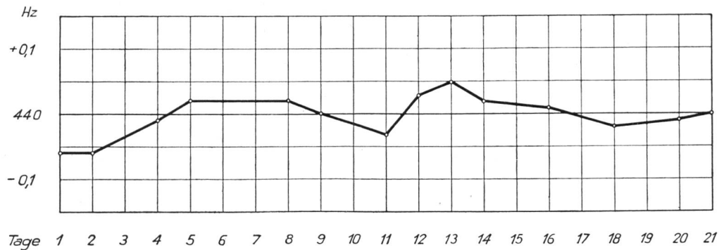
Fig. 5. Dauerversuch der Frequenzkonstanz. — Essai de durée de la fréquence.
