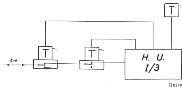
Fig. 1. Hauptumschalter I/3; zwei Apparate sind mit Vorschaltkästchen ausgerüstet
