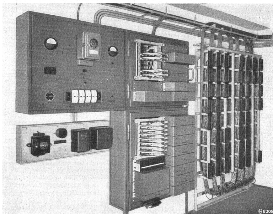
Fig. 8. Mit einem Vermittlerschrank zusammengeschalteter Hausautomat für maximal 90 automatische Hausanschlüsse. Einschleifen-Rückfrage-System. Rechts vom Automat der Hauptverteiler
