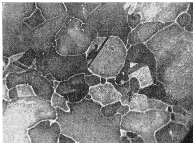
Fig. 3. Gefüge der Innenfläche des Bleimantels
