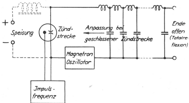
Fig. 2. Impuls-Modulationsschaltung
