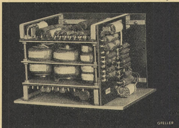
Elektrischer Filter, Innenansicht
