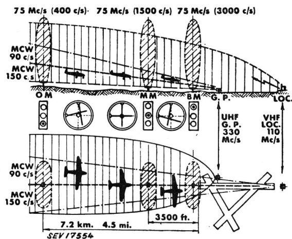
Fig. 7. Prinzipskizze der Blindlandanlage ILS Oben: Vertikale Leitebene des Bakensenders Unten: Horizontale Leitebene des Gleitwegsenders Mitte: Anzeige im Flugzeug
