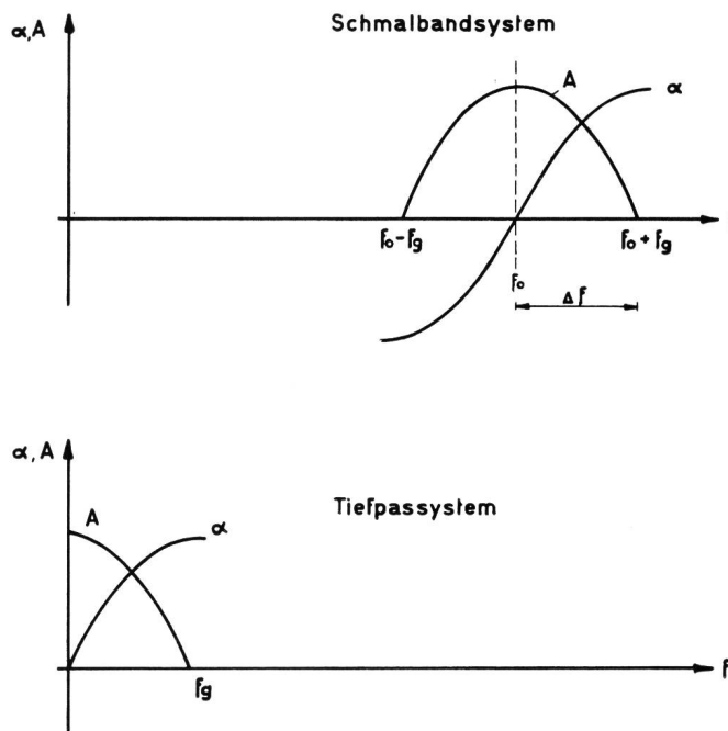
Fig. 4. Aequivalentes Tiefpaßsystem
