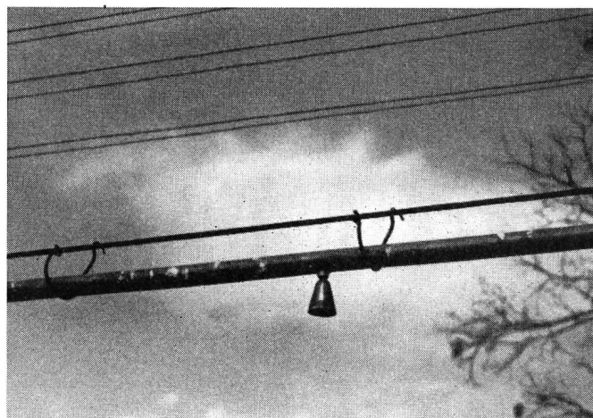
Fig. 22. Aération naturelle d'un câble aérien poreux
