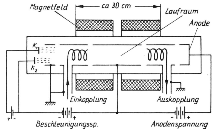
Fig. 25. Schema einer Doppelstrahlröhre
