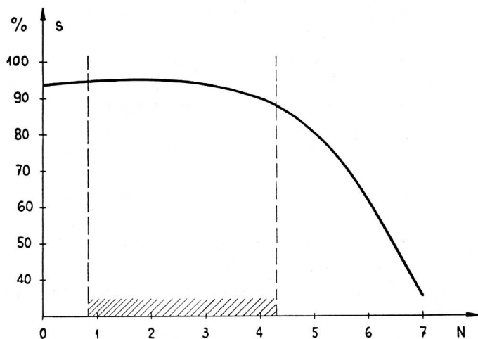
Fig. 3. Lautverständlichkeit einer Telefonverbindung mit neuen Stationen
