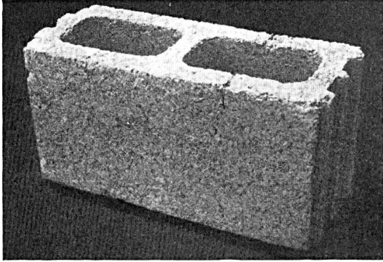
Fig. 3a. «Durisol»-Hohlkammersteine als Helmholtzresonatoren. Hohlkammerstein allein Briques creuses «Durisol» utilisées comme résonateurs de Helmholtz. Brique originale
