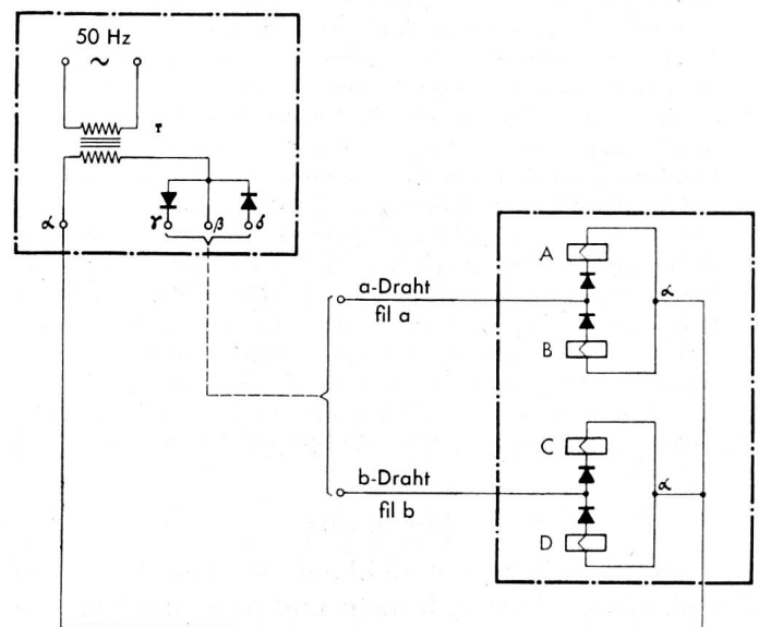
Fig. 1. Prinzip des Wählvorganges mittels Halb- und Ganzwellen Principe de la sélection au moyen de demi-périodes et de périodes entières
