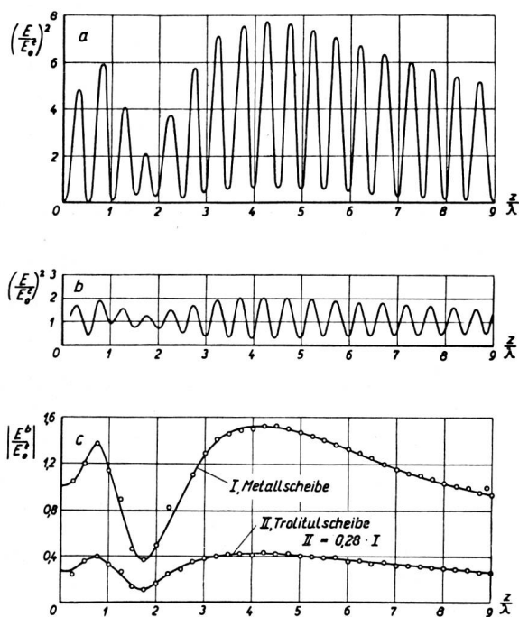
Fig. 7. Gemessenes relatives Amplitudenquadrat der elektrischen Feldstärke auf der Mittelnormale vor a) einer kreisförmigen Metallscheibe, Durchmesser d = 4\lambda b) einer Trolitulscheibe gleicher Grösse, Reflexionsfaktor r = 0,28 Aus a) und b) errechneter (o) Amplitudenverlauf der Beugungswelle
