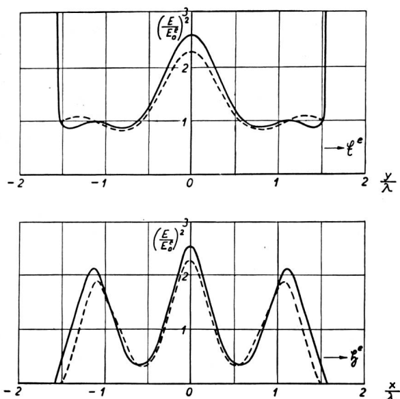
Fig. 2. Relatives Amplitudenquadrat der elektrischen Feldstärke in einer kreisförmigen Öffnung längs des zu \xi^e und \xi^e parallelen Durchmessers strenge Rechnung d = 3,18 \lambda (Andrejewski) gemessen d = 3 \lambda (Andrews)
