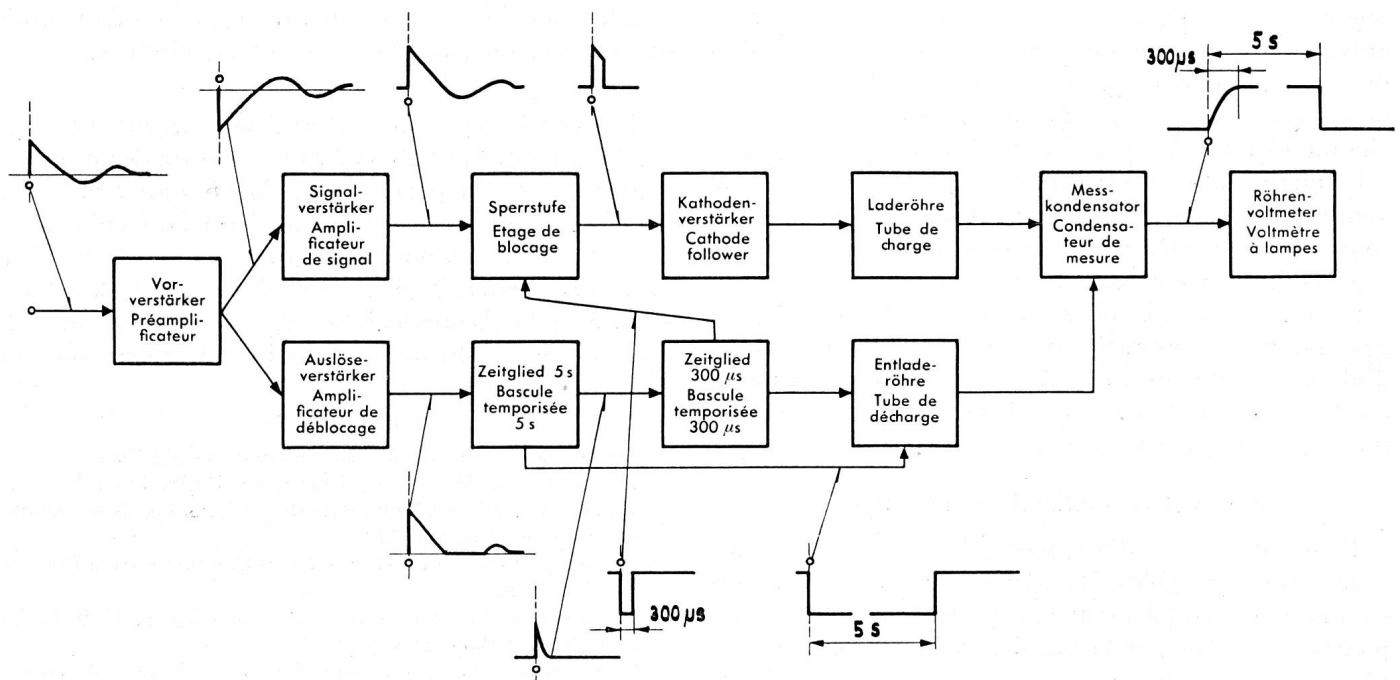
Fig. 1. Blockschema des Knackmessgerätes. Die Aufgabe der einzelnen Stufen ist aus dem Text ersichtlich
