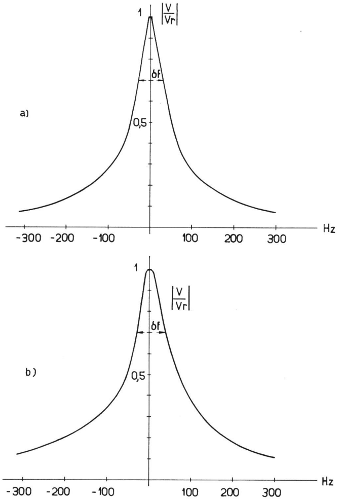
Frequenzabweichung von der Resonanzlage Fig. 26. Im Empfänger gemessene Selektivität des Empfängerkreises I a = mit L = 16 mHy; f_r = 8000 Hz; \delta f = 60 Hz; Q_{eff} = 133 b = mit L = 25 mHy; f_r = 8000 Hz; \delta f = 70 Hz; Q_{eff} = 115
