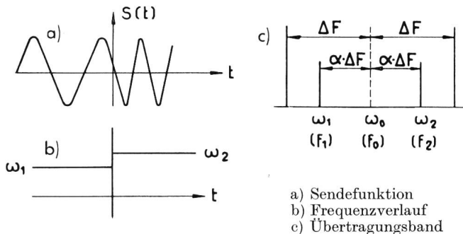
Fig. 3. Sprungfunktion bei der Frequenzmodulation und Lage der Frequenzen im Übertragungsband eines idealen Bandpasses.
