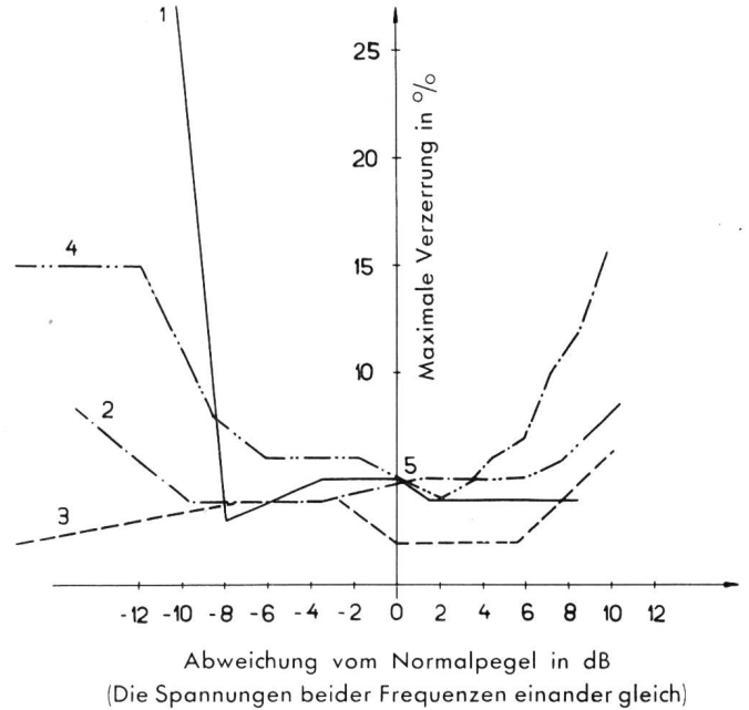
Fig. 29. Gemessene Verzerrungen in Funktion der Pegelschwankungen
