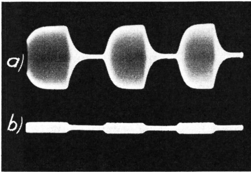
Fig. 24a. Ein- und Ausschwingvorgang im Empfängerkreis a) entspricht Fig. 23 c. \omega = \Omega = 8000 Hz (Signalfrequenz gleich der Resonanzfrequenz) (Impulslänge 20 ms) b) entspricht Fig. 24. |\omega - \Omega| = 300 Hz (Signalfrequenz weicht von der Resonanzfrequenz ab) \omega = 8000 Hz \Omega = 8300 Hz
