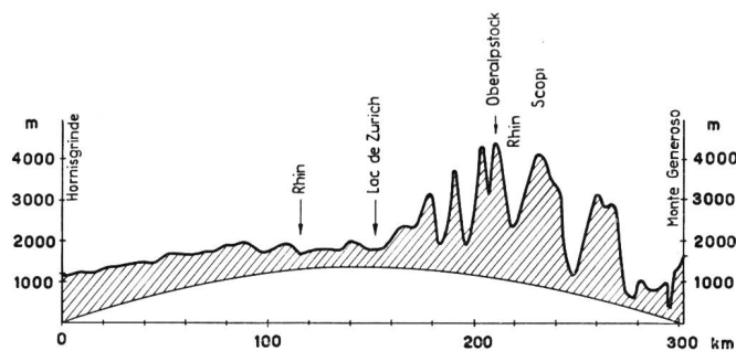
Fig. 1e. Profil Hornisgrinde-Monte Generoso. Surélévation 20:1
