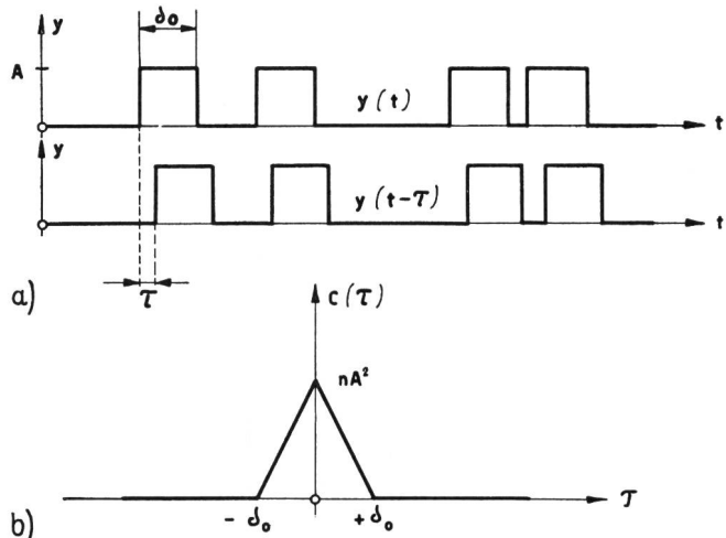
Fig. 33. Bildung der Autokorrelationsfunktion einer Folge identischer Impulse
