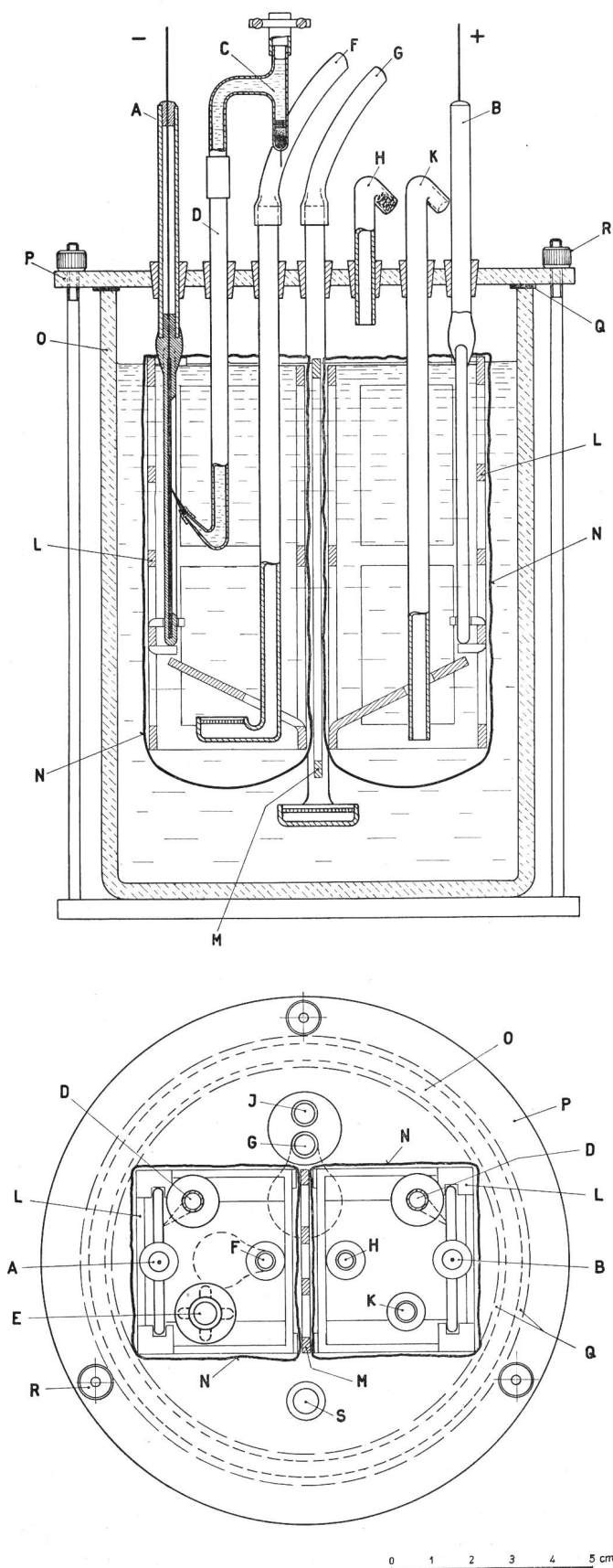
Fig. 9. Versuchs-Zelle für die kathodische Polarisation: A Bleikathode, B Platinanode, C Kalomel-Bezugselektrode, D Sonde zur Kalomelektrode, E Glasrührer, F Gaszu- führung für Kathodenraum, G Gaszuführung für Zwi- schenraum, H Gasausgang (mit Wattepfropfen), J Elek-
