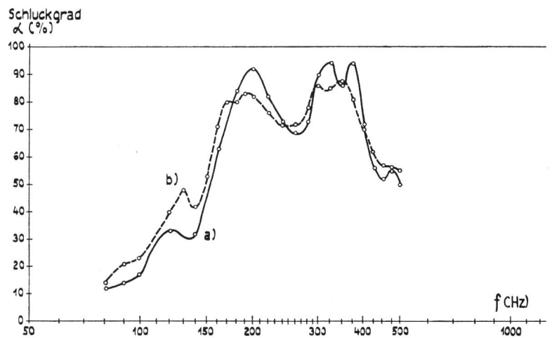
Fig. 7. Absorptionskurve der in Fig. 6 dargestellten Schlitzresonatoranordnung (Rohrmessung) a) ungedämpft b) Schlitz durch eine 10 mm starke Glaswattschicht schwach gedämpft
