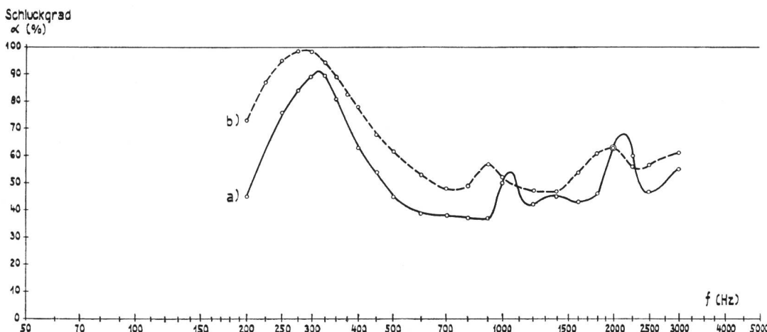
Fig. 3. 2 cm starke Akustikplatte mit 6 mm breiten Schlitz in 55 mm Abstand, vor einem 6 cm tiefen Luftpolster a) ohne Dämpfung b) gedämpft durch 2 cm Glaswolle hinter den Schlitz
