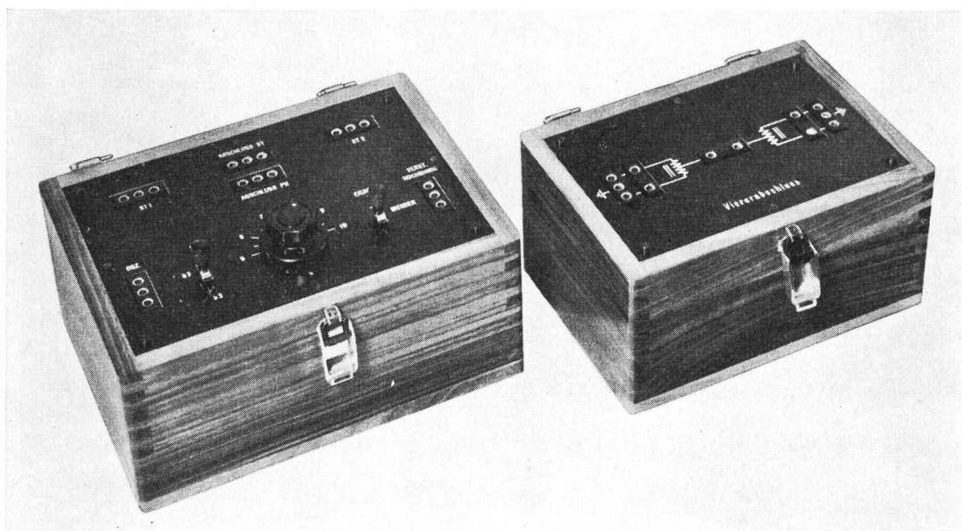
Fig. 4. Nebensprechmesser und Viererschluss
