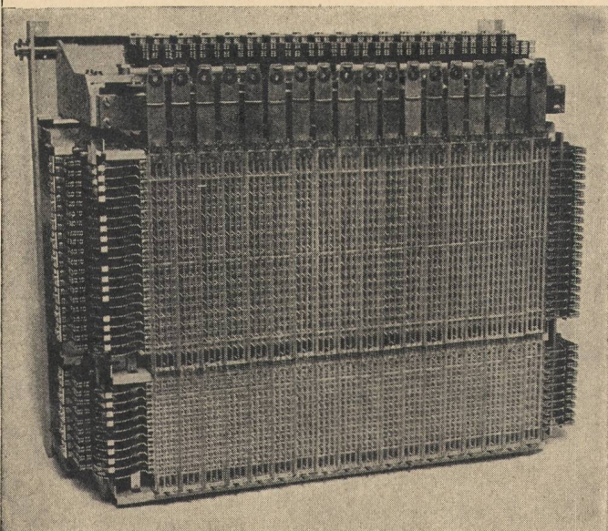
Kreuzwähler K 53
