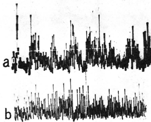
Fig. 19. Comparaison des oscillogrammes relevés à la sortie basse fréquence d'un récepteur CISPR captant a) le champ de la ligne Mühleberg-Laufenburg excitée par 6 générateurs à arc et b) le champ de la ligne 220 kV Mühleberg-Riddes en service normal ( f = 1400 \text{ kHz} , d = 50 \text{ m} ) Vergleich von Oszillogrammen, die am Niederfrequenzausgang des CISPR-Empfängers aufgenommen wurden. Der Empfänger erfasste hierbei a) das Störfeld der Leitung Mühleberg-Laufenburg bei Erregung durch 6 Funkengeneratoren und b) das Störfeld der 220-kV-Leitung Mühleberg-Riddes bei normalem Betrieb ( f = 1400 \text{ kHz} , d = 50 \text{ m} )
