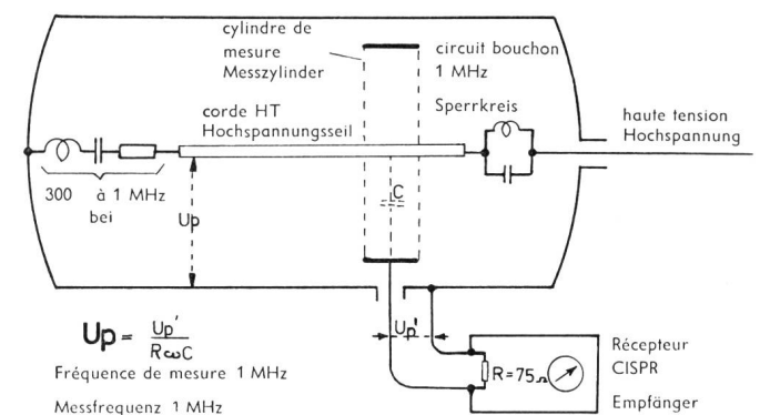
Fig. 16. Enceinte climatique pour la mesure du pouvoir perturbateur d'échantillons de conducteurs de ligne Klimareuse zur Messung des Störvermögens an Versuchsmustern von Hochspannungsleitern
