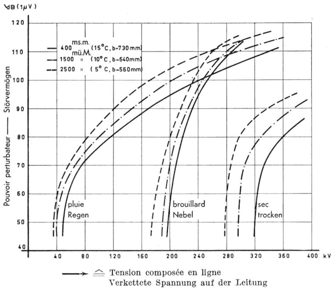
Fig. 17. Pouvoir perturbateur d'un conducteur Aldrey de 30,6 mm de diamètre mesuré en nasse sous pluie avec brouillard et à sec à 3 «altitudes» Störvermögen eines Aldrey-Seiles von 30,6 mm Ø, gemessen in der Reuse bei Regen, Nebel und trocken in drei «Höhenlagen»
