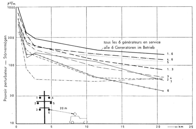
Fig. 23. Champ magnétique le long de la ligne Mühleberg-Laufenburg avec excitation à Niederoesch (à la fréquence de 1500 kHz et à 20 m de distance)
