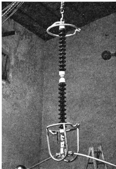
Fig. 15. Pouvoir perturbateur d'une chaîne d'isolateurs pour ligne à 220 kV avec corbeille de protection type EWZ Störvermögen einer Isolatorenkette für 220-kV-Leitungen mit Schutzkorb Typ EWZ
