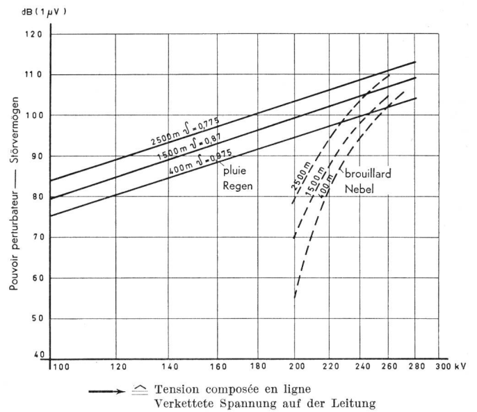
Fig. 17a. Effet de la tension relative de l'air \delta et de la tension de service U_L sur le pouvoir perturbateur U_p d'un échantillon de conducteur de \varnothing = 30,6 mm
