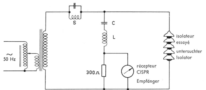
Fig. 13. Dispositif de mesure du pouvoir perturbateur des isolateurs à 1 MHz Messeinrichtung für das Störvermögen von Isolatoren bei 1 MHz
