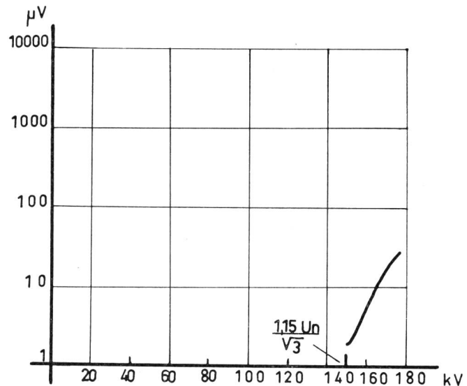
Fig. 15. Pouvoir perturbateur d'une chaîne d'isolateurs pour ligne à 220 kV avec corbeille de protection type EWZ Störvermögen einer Isolatorenkette für 220-kV-Leitungen mit Schutzkorb Typ EWZ
