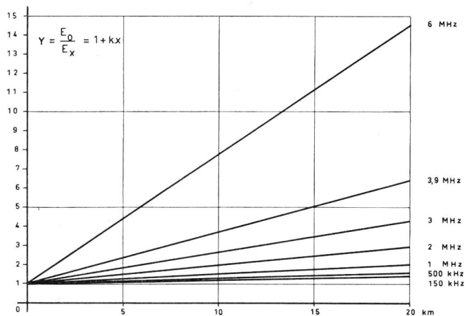
Fig. 25. Rapport entre le champ E_0 mesuré près des générateurs et le champ E_x mesuré à une distance x le long de la ligne. Verhältnis zwischen der Feldstärke E_0 - gemessen in Nähe der Störgeneratoren - und der Feldstärke E_x - gemessen bei einer Distanz x längs der Leitung
