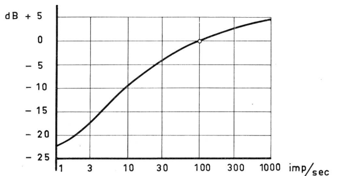
Courbe de réponse aux impulsions brèves répétées régulièrement Wiedergabekurve bei kurzen, regelmässig wiederholten Impulsen
