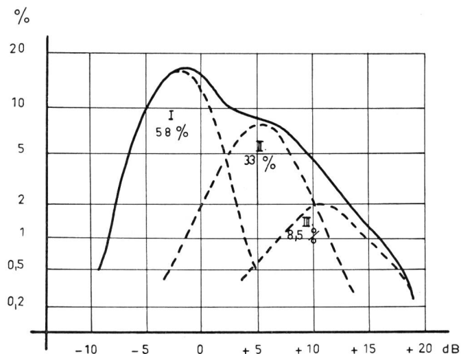
Fig. 12. Exemple d'analyse d'une répartition statistique Répartition moyenne des fréquences statistiques observées à Grund et Brunnen pour une largeur de classe de 2 dB
