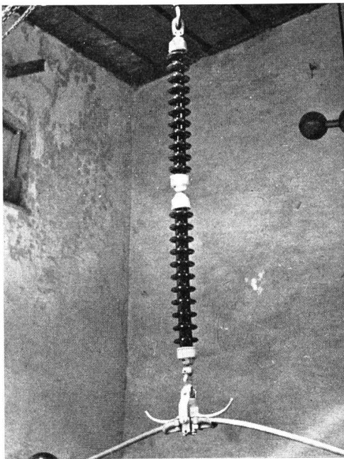
Fig. 14. Pouvoir perturbateur d'une chaîne d'isolateurs pour ligne à 220 kV avec pince à cornes et conducteur Aldrey 550 \text{ mm}^2 Störvermögen einer Isolatorenkette für 220 kV-Leitungen mit Seilklemme mit Hörnern und Aldrey-Seil 550 \text{ mm}^2
