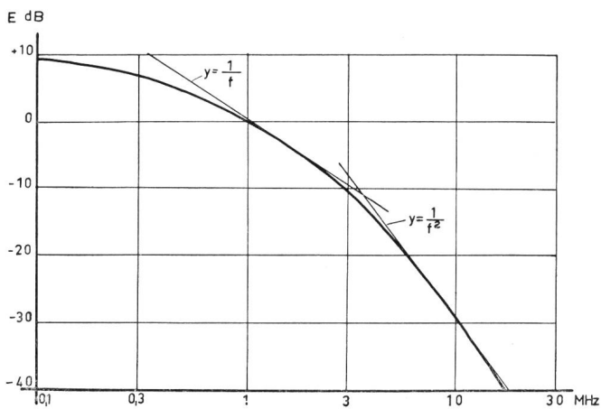
Fig. 6. Spectre typique relevé sous les lignes à haute tension longues. Ce spectre est pratiquement identique à celui d'impulsions de forme U_t = k (e^{-2,2 \cdot 10^6 t} - e^{-21 \cdot 10^6 t}) Typisches Spektrum, aufgenommen unter langen Hochspannungsleitungen. Dieses Spektrum ist praktisch identisch mit demjenigen von Impulsen von der Form: U_t = k (e^{-2,2 \cdot 10^6 t} - e^{-21 \cdot 10^6 t})
