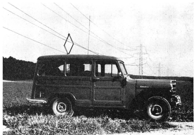
Fig. 7. Voiture de mesure équipée d'un récepteur CISPR avec cadre et antenne tige Messwagen, ausgerüstet mit einem CISPR-Empfänger mit Rahmen- und Stabantenne
