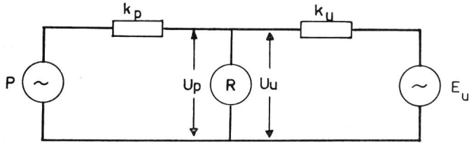
Fig. 3. Eléments d'un cas de perturbation Im Störungsfall beteiligte Elemente
