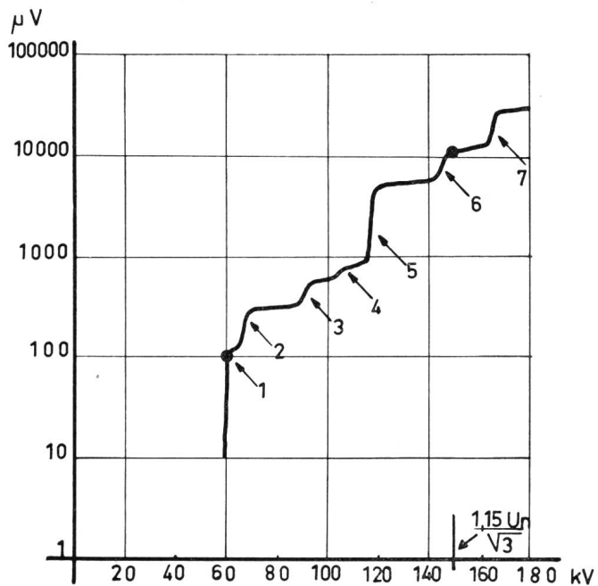
Fig. 14. Pouvoir perturbateur d'une chaîne d'isolateurs pour ligne à 220 kV avec pince à cornes et conducteur Aldrey 550 \text{ mm}^2 Störvermögen einer Isolatorenkette für 220 kV-Leitungen mit Seilklemme mit Hörnern und Aldrey-Seil 550 \text{ mm}^2
