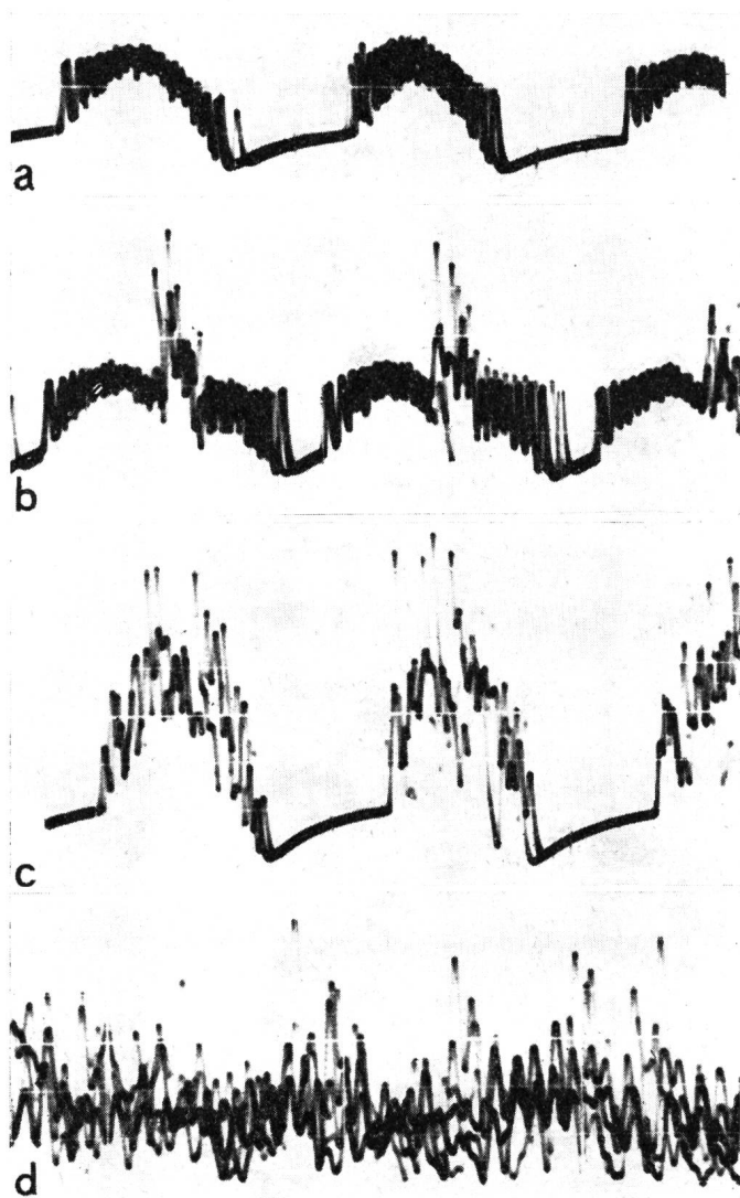
Fig. 21. Oscillogrammes obtenus avec le dispositif de la fig. 20 a) 1 générateur excité par la phase R b) 1 générateur excité par chacune des phases R et S c) 2 générateurs excités par la phase R d) 2 générateurs excités par chacune des phases R, S, et T
