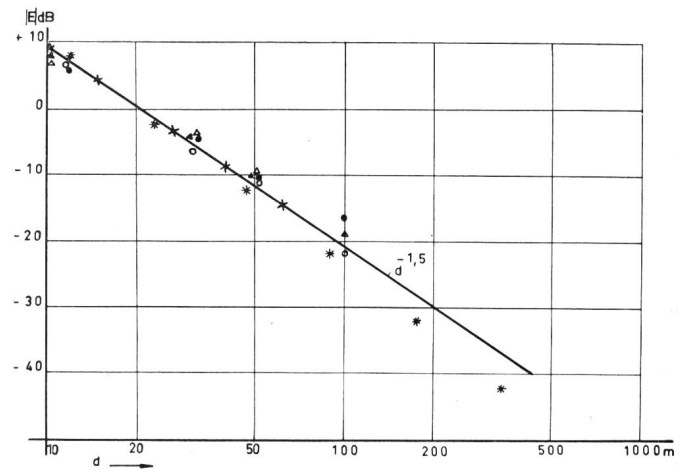
Fig. 5. Décroissance du champ perpendiculairement à la ligne x moyenne de 82 mesures américaines ( d^{-1,5} ) * mesures suédoises ( d^{-1,7} ) ● 220 kHz à 2,7 km des sources ( d^{-1,25} ) Ligne 220 kV ○ 1500 kHz à 2,7 km des sources ( d^{-1,5} ) Mühleberg- ▲ 220 kHz à 11,2 km des sources ( d^{-1,4} ) Laufenburg △ 1500 kHz à 11,2 km des sources ( d^{-1,25} ) Abnahme des Feldes quer zur Leitung x Mittelwert aus 82 amerikanischen Messungen ( d^{-1,5} ) * Schwedische Messungen ( d^{-1,7} ) ● 220 kHz in 2,7 km Distanz von den Quellen ( d^{-1,25} ) ○ 1500 kHz in 2,7 km Distanz von den Quellen ( d^{-1,5} ) ▲ 220 kHz in 11,2 km Distanz von den Quellen ( d^{-1,4} ) △ 1500 kHz in 11,2 km Distanz von den Quellen ( d^{-1,25} ) Leitung Mühleberg-Laufenburg
