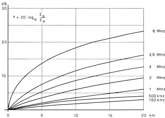
Fig. 24. Atténuation totale le long de la ligne 220 kV Mühleberg-Laufenburg en fonction de l'éloignement de la source. Gesamtdämpfung längs der 220-kV-Leitung Mühleberg-Laufenburg in Funktion der Entfernung von der Störquelle
