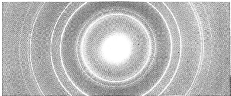
Fig. 4. Elektronenbeugungsdiagramm der in der Figur 3 abgebildeten Aufdampfschicht. Interferenzen des metallischen Bleis
