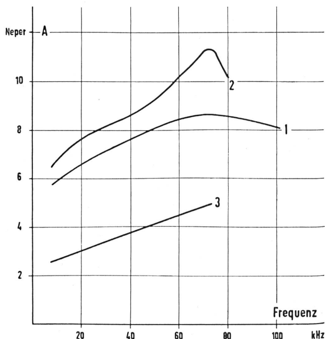
Fig. 8. Phantomdämpfung einer Sperrspulenschaltung und des zugehörigen Verstärkerfeldes Affaiblissement fantôme d'un circuit de bobine de blocage et de la section d'amplification y relative
