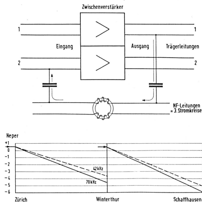
Fig. 2. (Oben) Die Entstehung des Sekundärnebensprechens bei Zwischenverstärkung und dessen Dämpfung mit Sperrspulen
