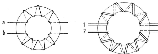
Fig. 4. (links) Stammsperrspule, für Schlaufe a-b nicht induktiv (à gauche) Bobine de blocage de base, pour lacet a-b non inductif
