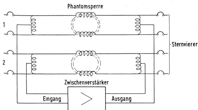
Fig. 3. Anschaltung des Phantoms an den Zwischenverstärker und Sperrung des durchgeschalteten Vierers für Trägerfrequenz
