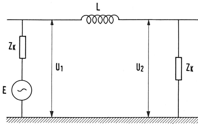
Fig. 5. Unsymmetrisch gestörter Stromkreis mit Sperrspule Circuit avec bobine de blocage dérangé asymétriquement
