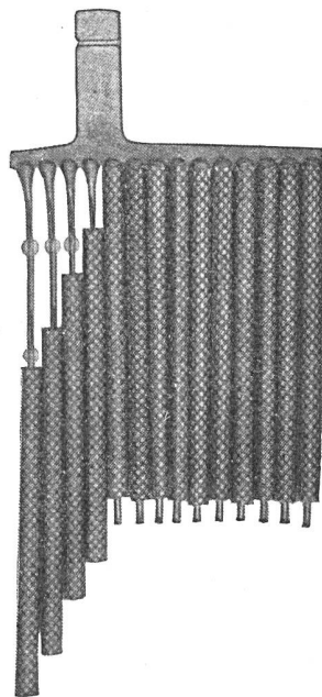
Fig. 14. Electrona-Dural-Platte (Gitter mit teilweise darübergeschobenen Kunststoffröhrchen, mit Glasseideschlauch im Innern)
