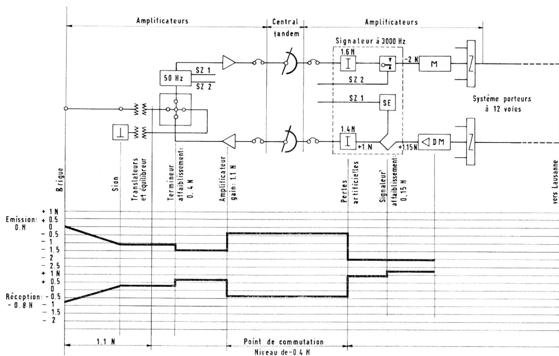
Fig. 11. Communication tandem Brig-Lausanne 2 fils - 4 fils
