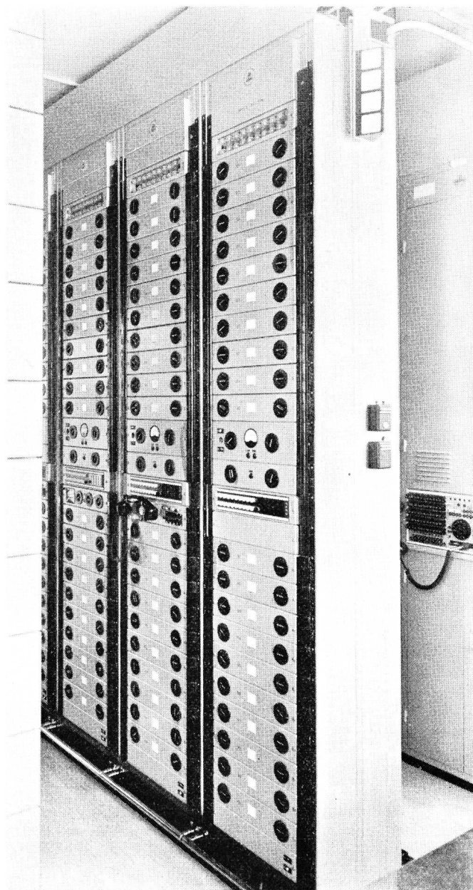
Fig. 14. Vue partielle des bâtis d'amplificateurs
