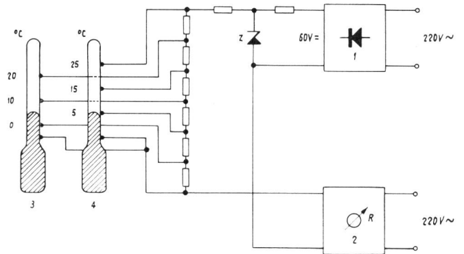
Fig. 1. Kontaktthermometer
