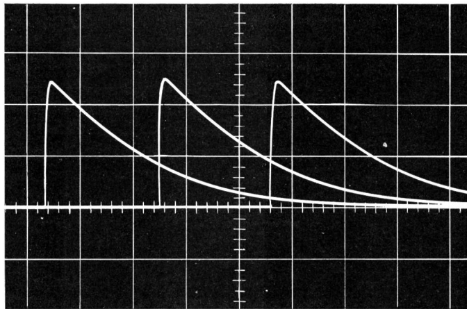
Fig. 2. Oszillogramm eines «Lettalite»-Phosphors Oscillogramme d'un produit phosphorescent «Lettalite»
