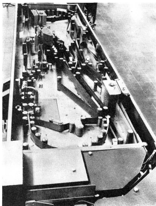
Fig. 9. Aufstellmaschine der Firma Telefunken Machine à redresser de la maison Telefunken
