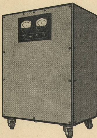
MA 28-125 (18-36V/125A)
