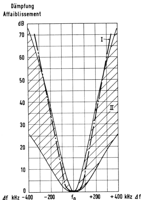
Fig. 8. Statische Selektivität
