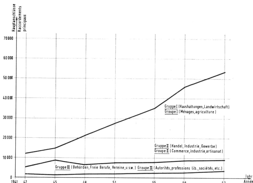
Fig. 9b. Augmentation annuelle des raccordements principaux par catégorie Jährliche Zunahme der Hauptanschlüsse nach Wirtschaftsgruppen
