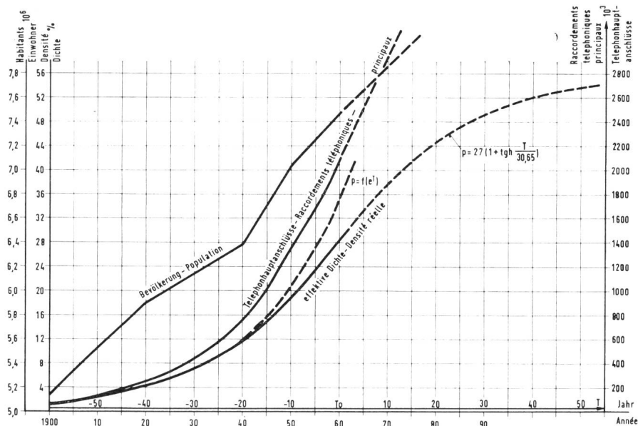
Fig. 6. Développement du téléphone en Suède Entwicklung des Telefons in Schweden
