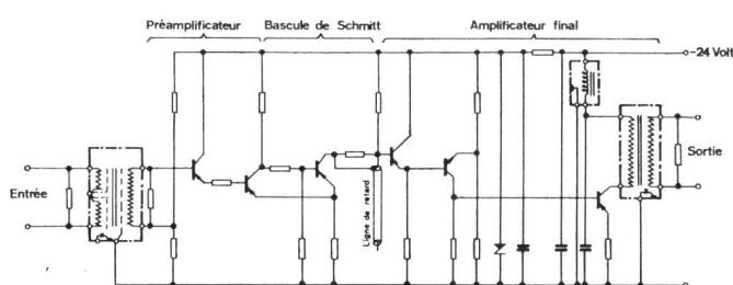
Fig. 4 Générateur d'harmoniques
