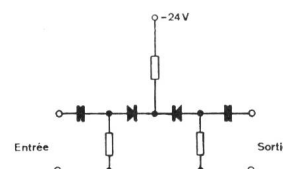
Fig. 5 Limiteur
