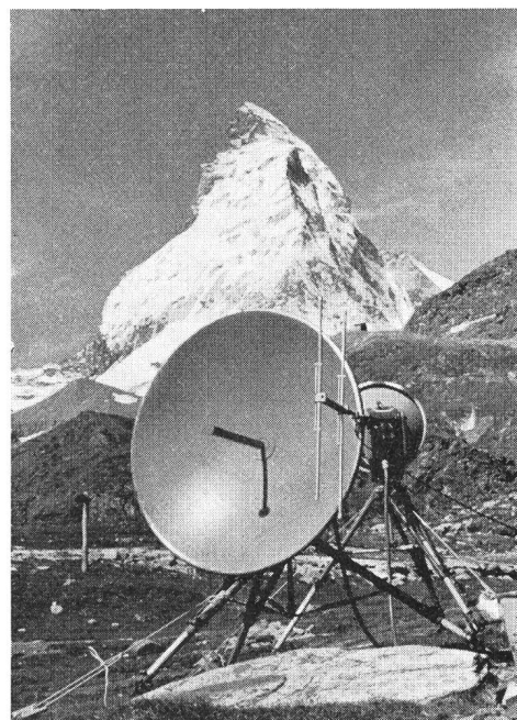
Fig. 8 Schwarzsee: 7-GHz-Bildverbindung mit Hörnli und Gornergrat (vorne)
