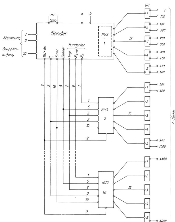
Fig. 3 Verbindungsdiagramm Sender Diagramme de jonction de l'émetteur
