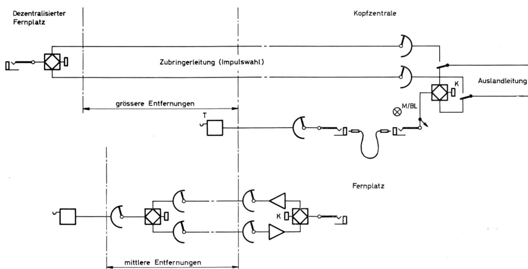
Fig. 5 Alte Durchschaltetechnik («Schnurverstärker» nicht dargestellt) – Ancienne technique de connexion (les «répéteurs sur cordons» ne sont pas représentés)
